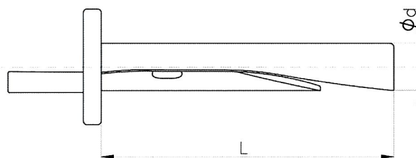
Rysunek A2. Łącznik rozporowy wbijany TDN
