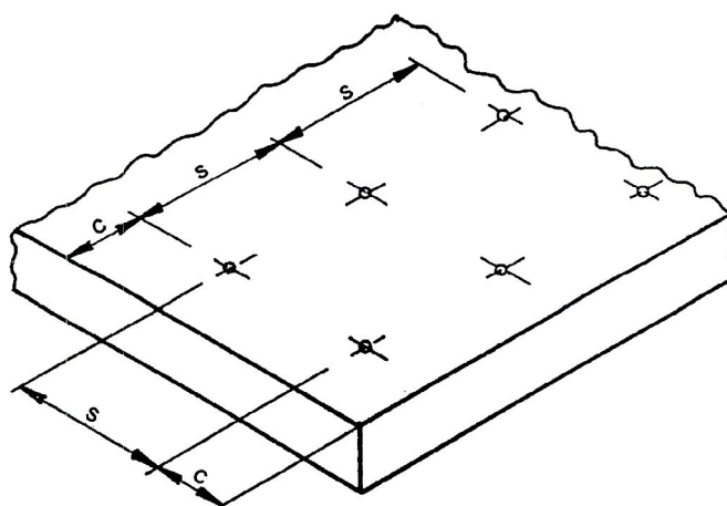
Rysunek B1. Parametry rozmieszczenia łączników rozporowych wbijanych SMM i TDN w podłożu s – rozstaw osiowy łączników, c – odległość łącznika od krawędzi podłoża
